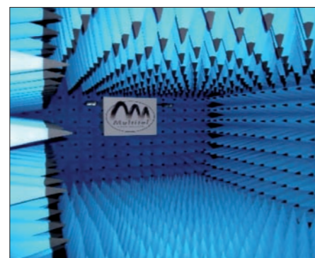
Figure : La chambre de MULTITEL est « full anéchoic » (le sol comporte aussi des mousses absorbantes)
